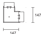
Spoj na dvije strane L Two-side connection L art.9470
