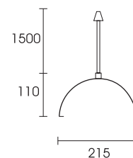
Rotirajuće vješanje na sajli Rotating suspension on a wire rope
