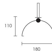
Plafonski rotirajući nosač Rotating ceiling carrier
