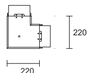
Spoj na dvije strane L Two-side connection L art.9471
