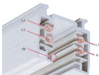
ELEKTRIFICIRANI KANAL L. 4000mm- TROFAZNO NAPAJSANJE ELECTRIFIED CONDUCTOR TRACK L. 4000mm- THREE-PHASE SUPPLY
